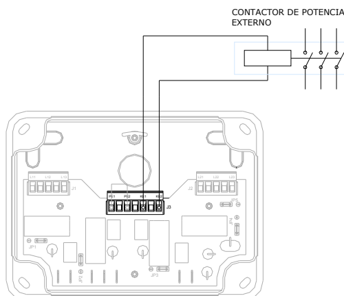
figura 6: Esquema de conexionado para uso de contactor externo.
