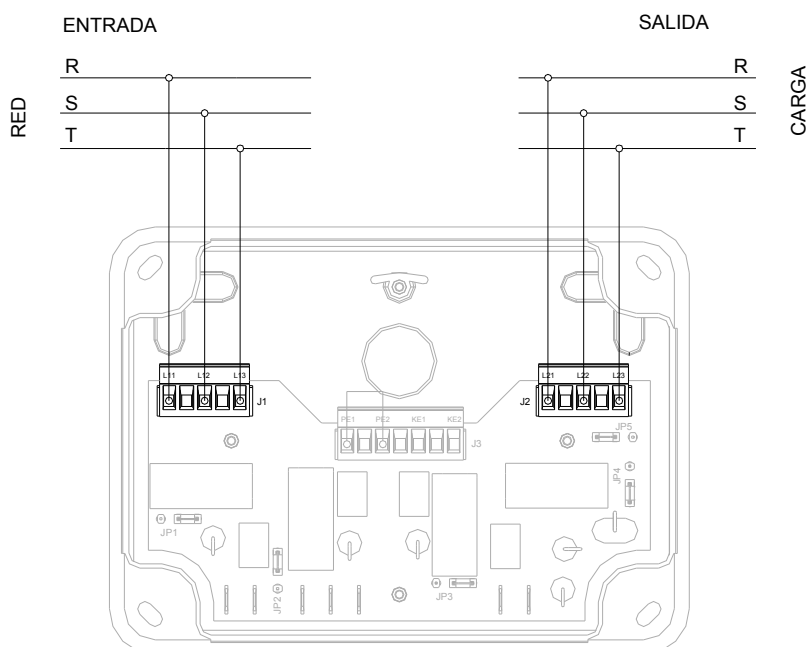
figura 1: Conexionado aplicación trifásica. Vista interior de la caja marcha-paro.
