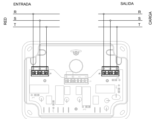
figure 2: Conexión entrada/salida para aplicación trifásica.
